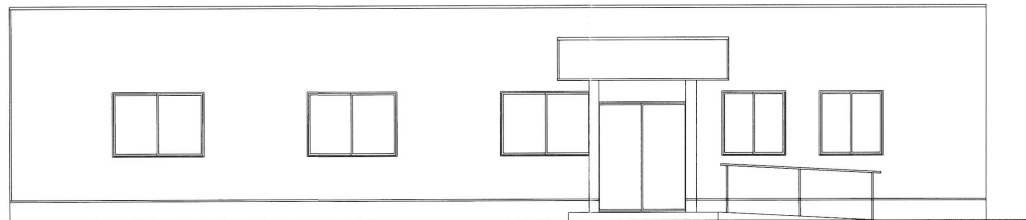
南立面図 S=1/100
